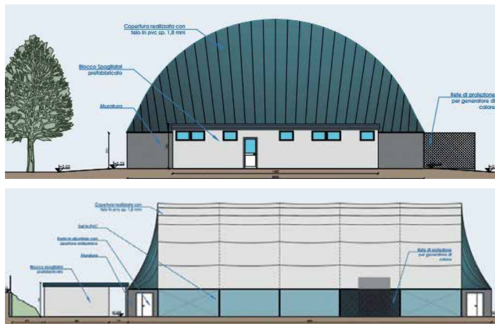
I due prospetti mostrano come verrà realizzata la nuova palestra della scuola primaria Falcone
