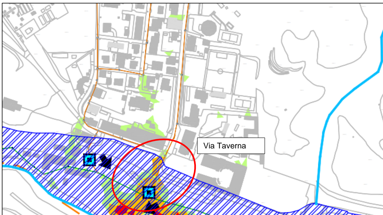
Figura 6: Aree con criticità idraulica dovute alla fognatura T50 in Via Taverna
