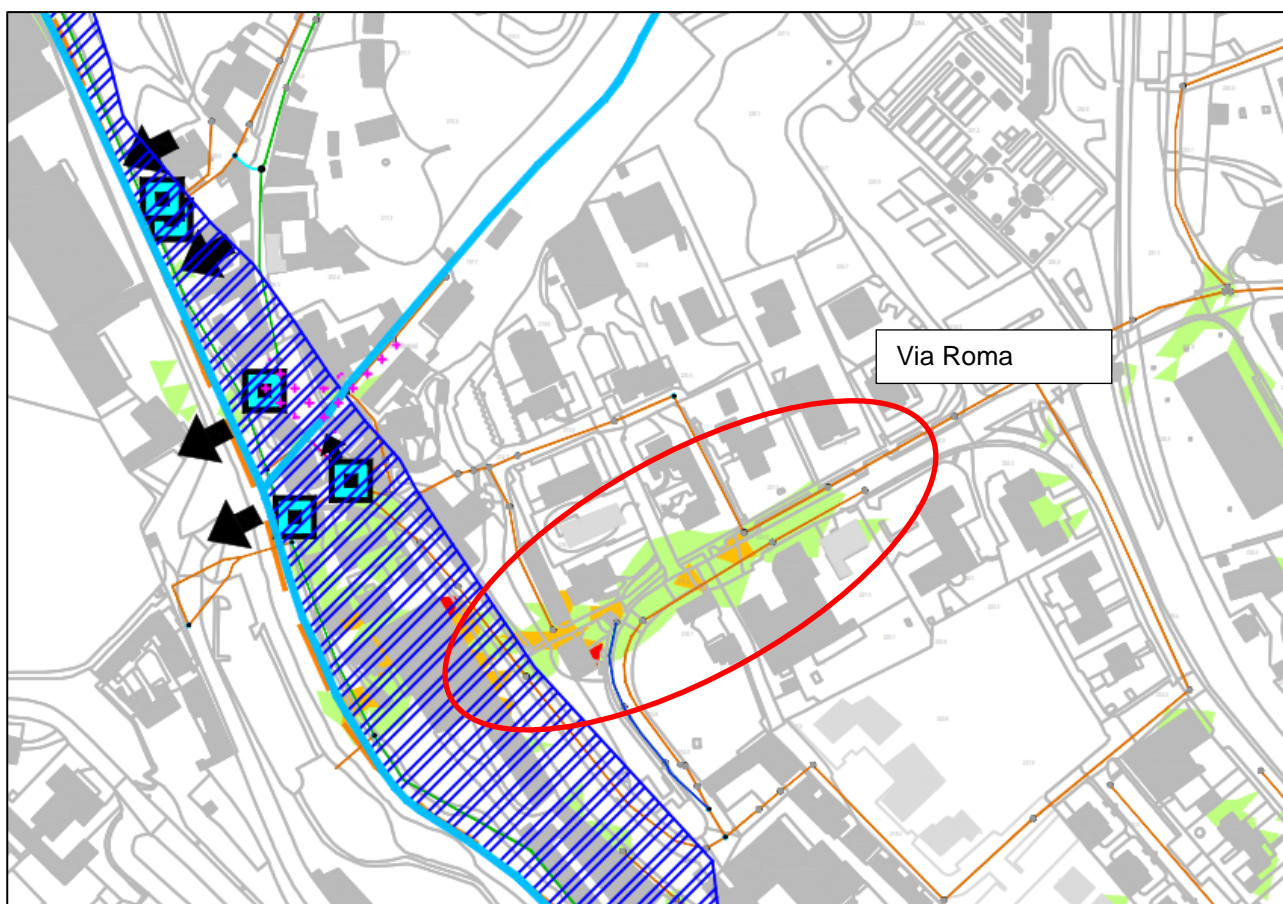
Figura 5: Aree con criticità idraulica dovute alla fognatura T50 in Via Roma
