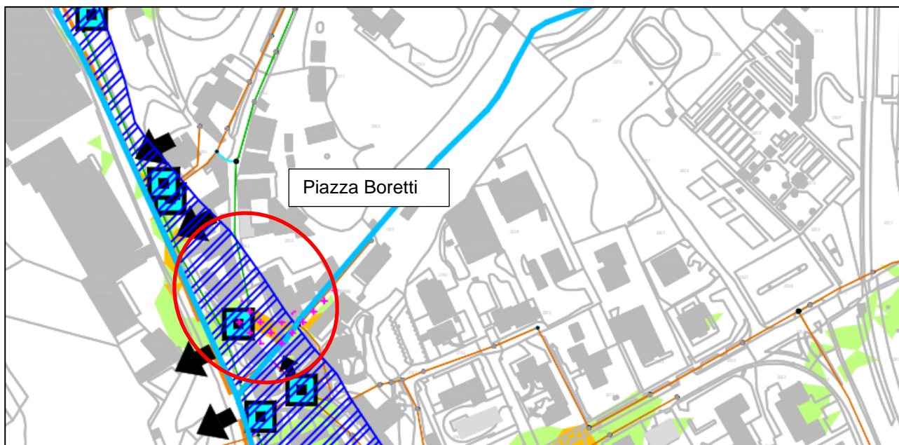
Figura 4: Aree con criticità idraulica dovute al reticolo idraulico T100 in Piazza Boretti
